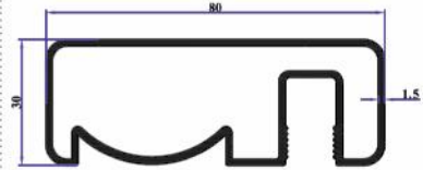
TA41 80x30 Küpeşte Profil 1,110 Kg/Mt
