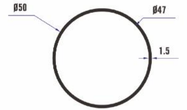
TA14 50x1,5 mm Profil 0,625 Kg/Mt
