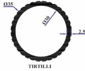
TA31 35x2,5 mm Tırtırlı Boru 0,637 Kg/Mt
