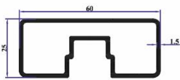
TA46 60x25 Ortadan Kanallı 0,780 Kg/Mt
