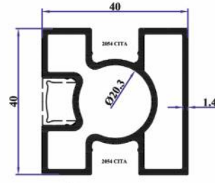
TA52 40x40 3 Kanallı Boru 0,890 Kg/Mt
