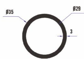
TA27 35x3 mm Profil 0,825 Kg/Mt
