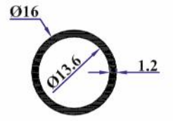
TA37 16x1,2 mm Boru 0,151 Kg/Mt
