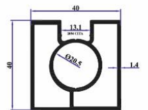
TA49 40x40 Tek Kanallı 0,895 Kg/Mt
