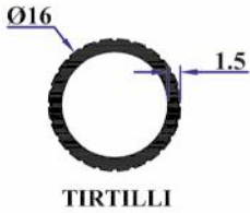
TA38 16x1,5 mm Tırtırlı Boru 0,175 Kg/Mt
