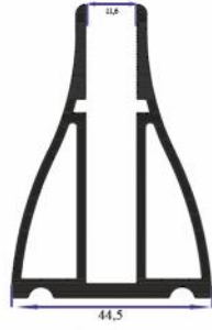
TA71 Mini Gemici 1,404 Kg/Mt
