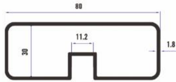
TA39 80x30 Cam Profil 1,122 Kg/Mt
