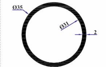
TA29 35x2 mm Boru 0,561 Kg/Mt
