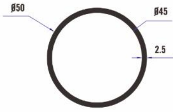
TA11 50x2,5 mm Profil 1,010 Kg/Mt
