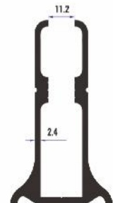
TA69 50'lik Alt Kızak Profil 1,755 Kg/Mt
