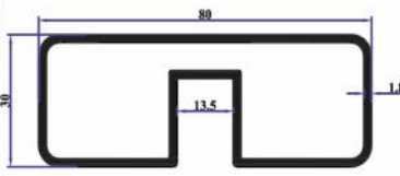
TA44 80x30 Ortadan Kanallı 1,193 Kg/Mt
