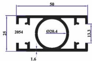
TA47 50x25 Dikme Profil 0,869 Kg/Mt
