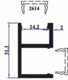
TA55 Takviyesiz Cam Tutucu 0,413 Kg/Mt
