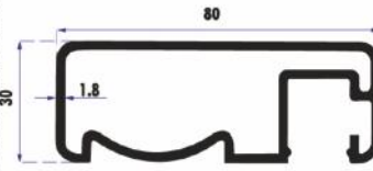
TA40 80x30 Küpeşte Profil 1,240 Kg/Mt
