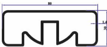
TA42 80x30 Ortadan Kanallı 1,147 Kg/Mt
