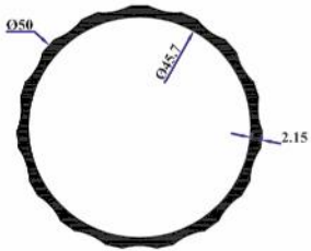
TA18 50'lik Tırtırlı Boru 0,730 Kg/Mt
