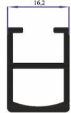
TA61 Cam Kızağı 0,285 Kg/Mt
