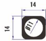
TA65 14x14 Kare Profil 0,255 Kg/Mt
