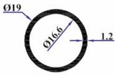
TA34 19x1,2 mm Boru 0,181 Kg/Mt
