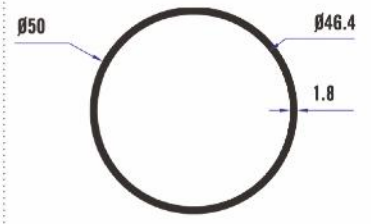
TA13 50x1,8 mm Profil 0,750 Kg/Mt
