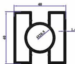
TA48 40x40 Çift Kanallı 0,890 Kg/Mt
