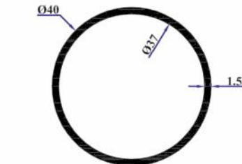
TA20 40x1,5 mm Boru 0,488 Kg/Mt
