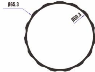
TA19 65'lik Tırtırlı Profil 1,100 Kg/Mt
