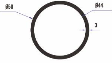
TA10 50x3 mm Profil 1,200 Kg/Mt
