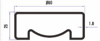
TA45 60x25 Kutu Profil 0,845 Kg/Mt
