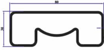
TA43 80x30 Profil 1,150 Kg/Mt
