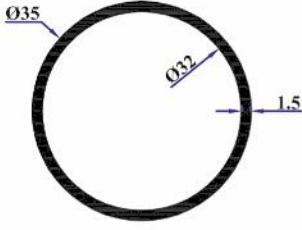
TA30 35x1,5 mm Boru 0,426 Kg/Mt
