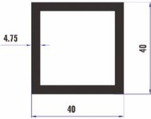
TA54 40x40 Kare Profil 2,350 Kg/Mt
