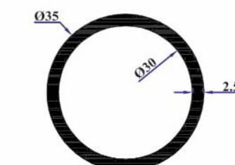
TA28 35x2,5 mm Boru 0,691 Kg/Mt
