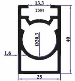
TA73 40x25 Tek Kanallı 0,774 Kg/Mt
